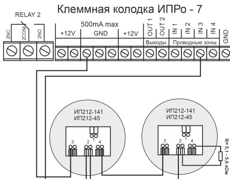
Подключение 2-х датчиков
