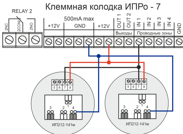
Подключение 2-х датчиков
