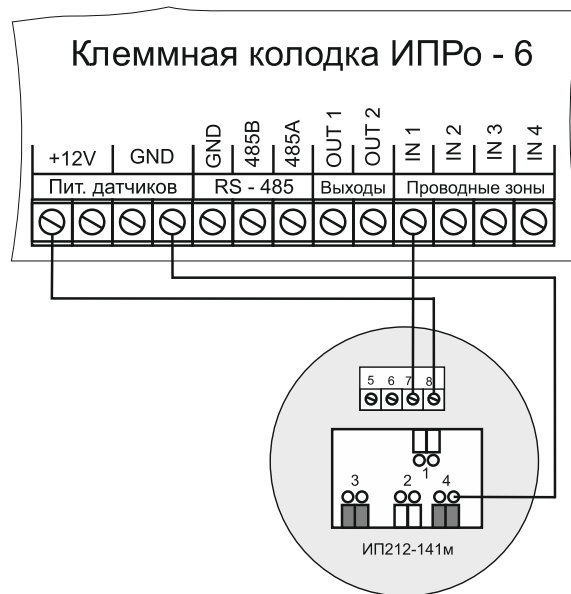
Подключение 1 датчика
