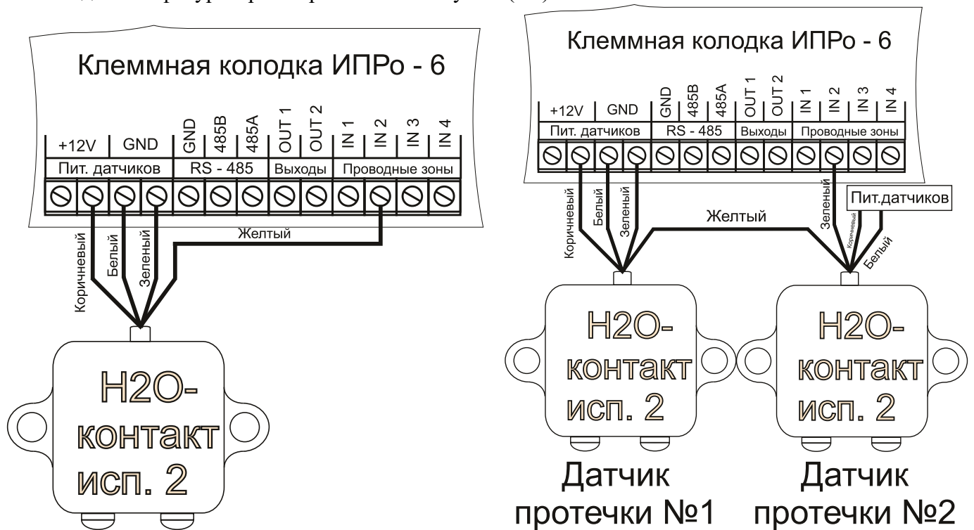
Подключение 1 датчика
