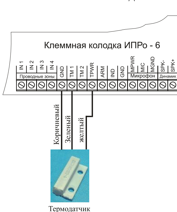
Подключение одного датчика
