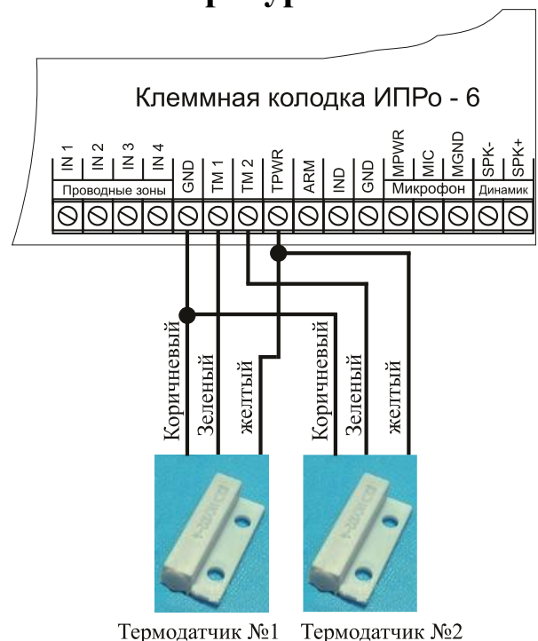
Подключения 2-х датчиков
