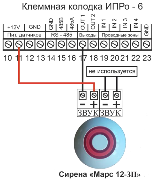
Подключение сирены «МАРС» или аналогичной с током потребления до 1А
