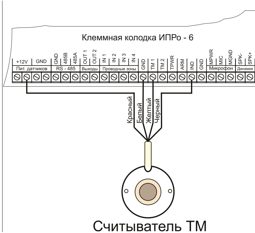
Считыватель с подсветкой 12В (внешний извещатель)
