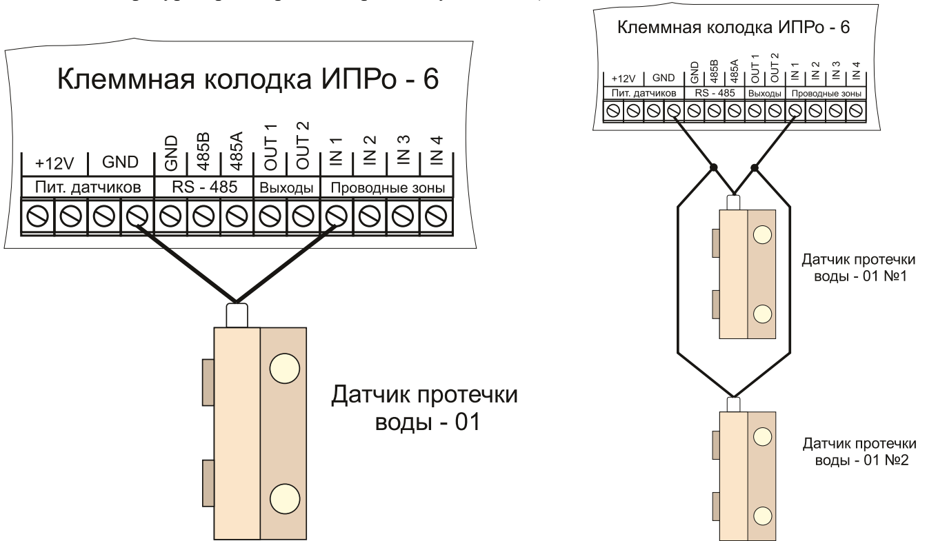
Подключение 1 датчика
