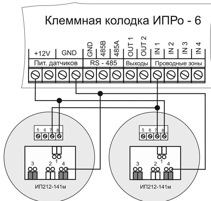
Подключение 2-х датчиков
