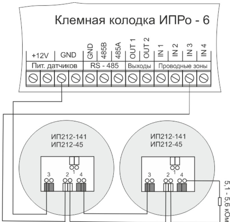
Подключение 2-х датчиков
