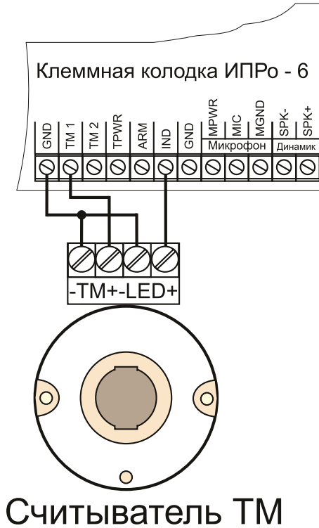
Считыватель с подсветкой 3,3В (светодиод)
