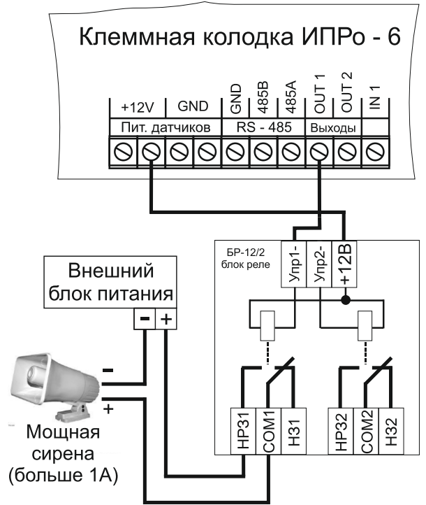
Подключение сирены с током потребления более 1А
